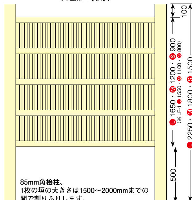
大垣加工寸法表
