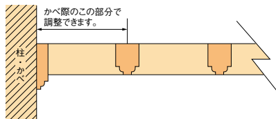
廻り縁 組手 (ワンタッチ加工)
