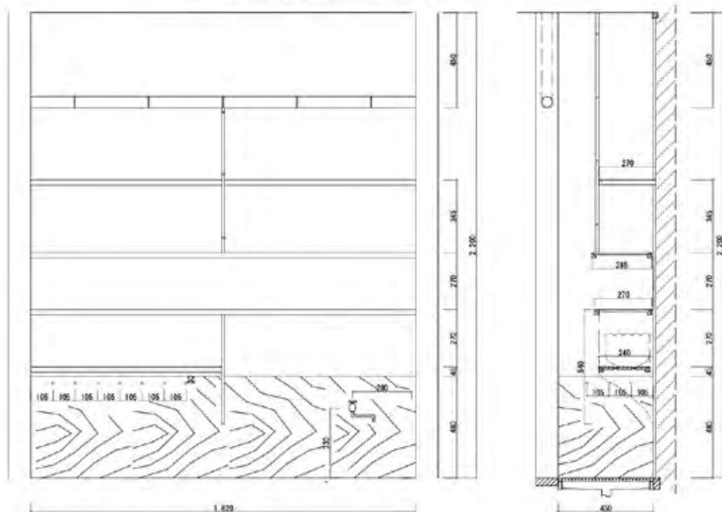
裏千家水屋（間口6尺）
