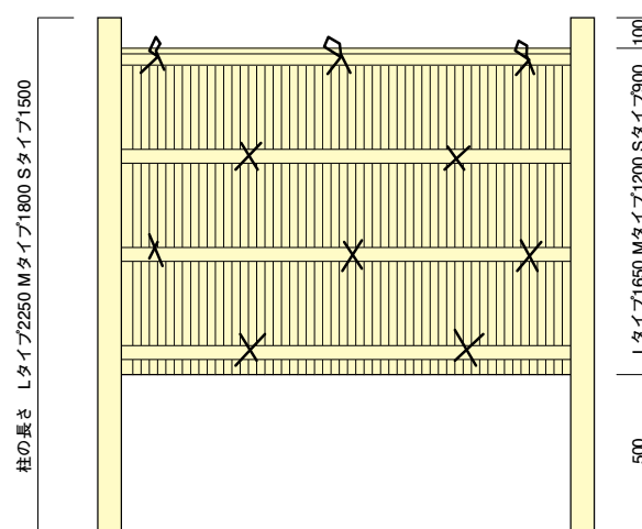
大垣加工寸法表
